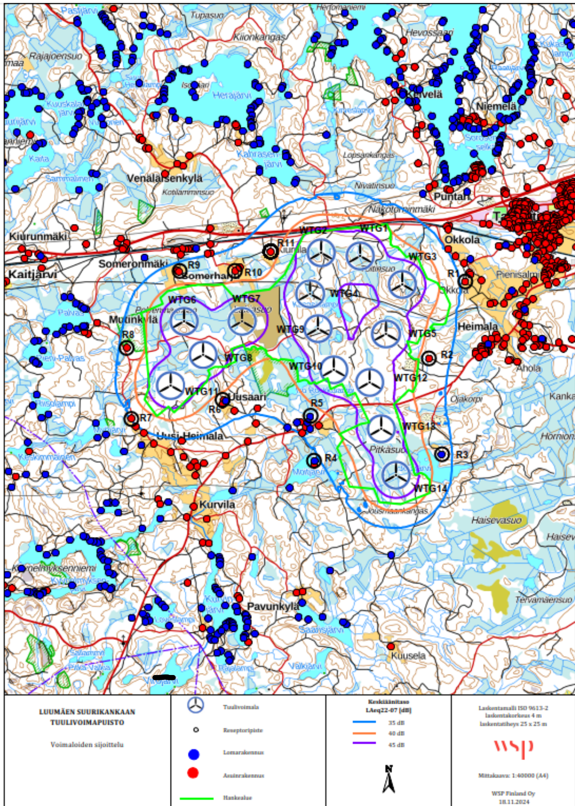
Kuva 6-43 Tuulivoimaloiden aiheuttamat melun keskikäänitason vyöhykkeet.
