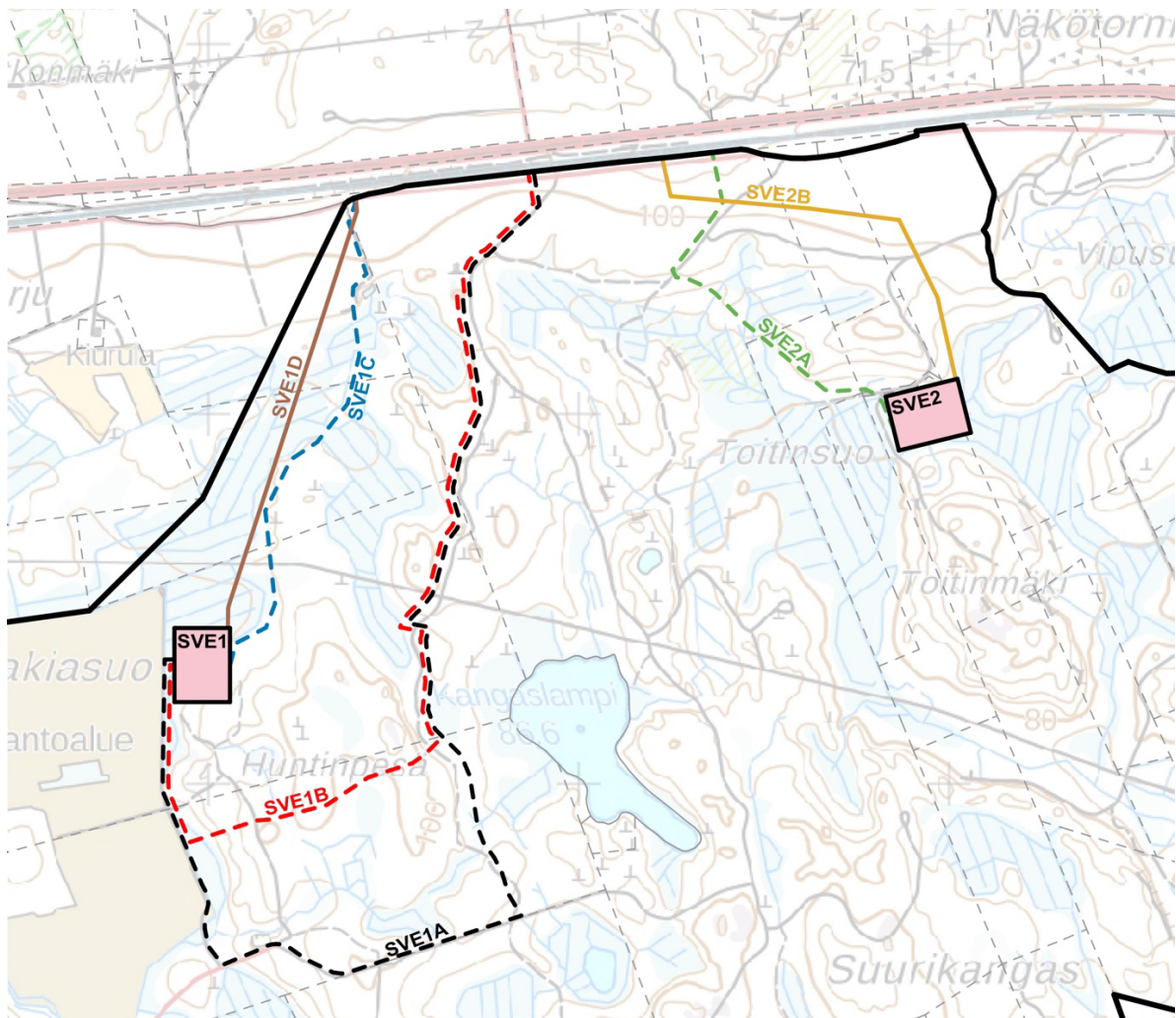
Kuva 5-1 Vaihtoehtoiset energiahuoltoalueet SVE1 JA SVE2 (kaavamerkintä EN) sekä vaihtoehtoiset sähkönsiirtoreitit kaava-alueella. Ehjällä viivalla esitetyt SVE1D ja SVE2B ovat ilmajohtoja ja katkoviivalla esitetyt SVE1A, SVE1B, SVE1C ja SVE2A ovat maakaapeleita.
