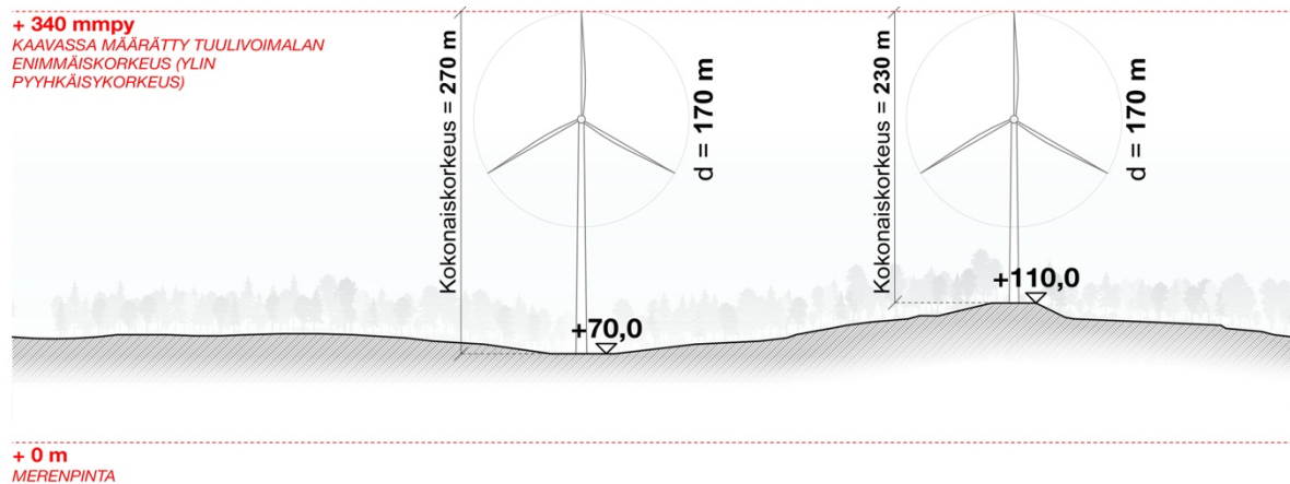
Kuva 7-2 Tuulivoimaloiden kokonaiskorkeuden rajoittuminen lentoesterajoituksen mukaan.
