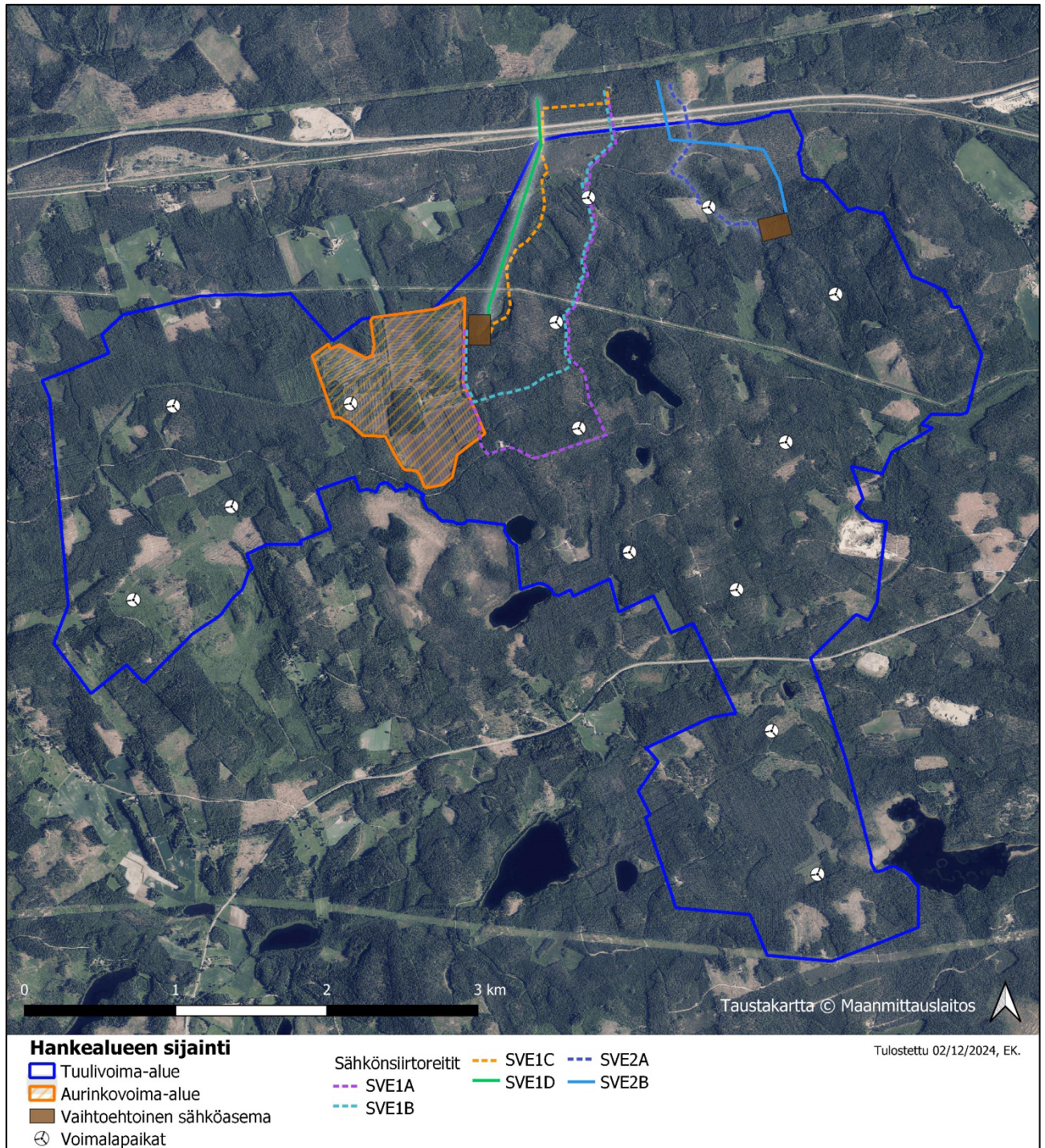
Kuva 6-8 Kaava-alue, voimalapaikat ja sähkönsiirtovaihtoehdot.
