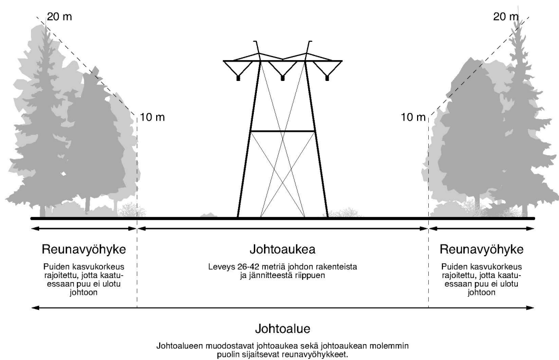
Kuva 7-5, 110 kV voimajohdon alustava tilantarve.
