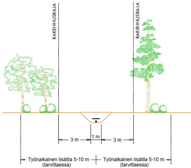
Kuva 7-4 Maakaapelin alustava tilantarve
