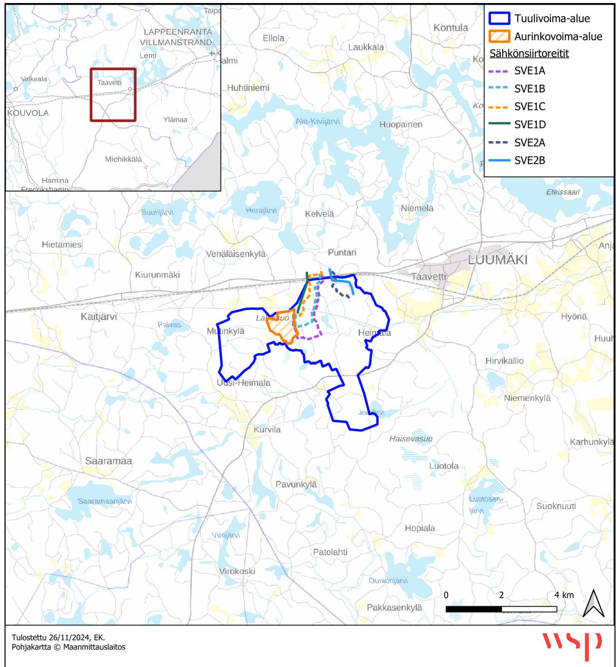
Kuva 1-1 Kaava-alueen sijainti ja sähkösiirtoreittien vaihtoehdot
