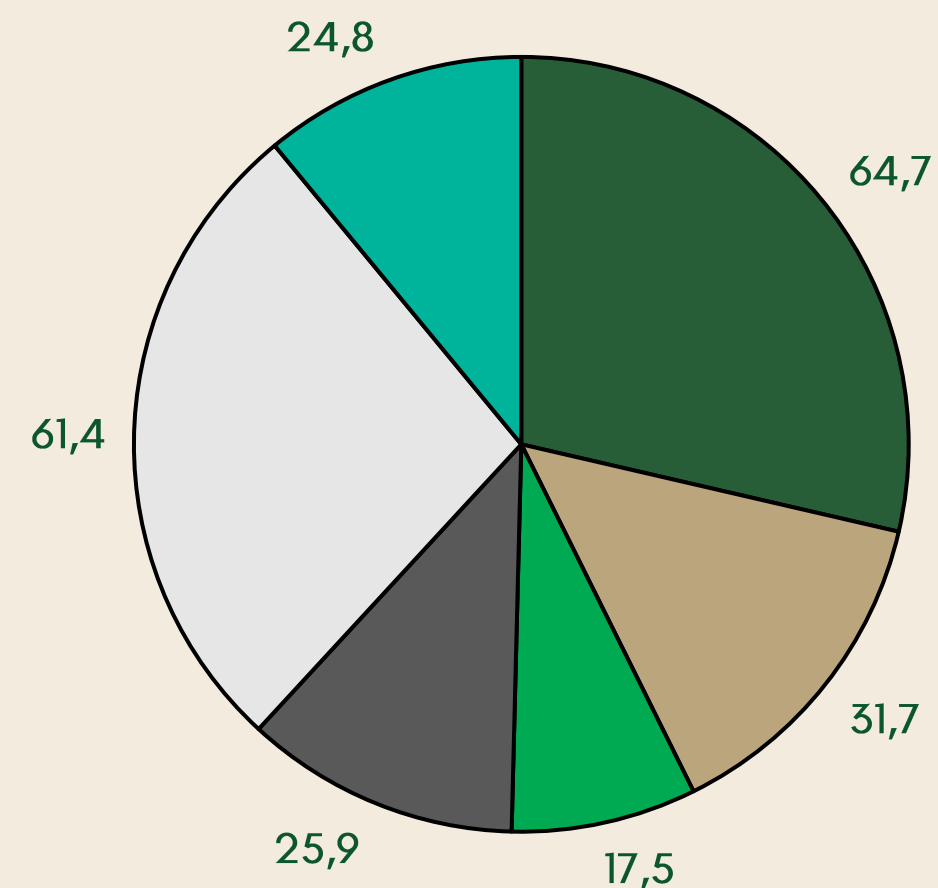
Energia 2021 Etelä-Karjala SYKE ALas-laskenta, päästöt ktCO 2e
