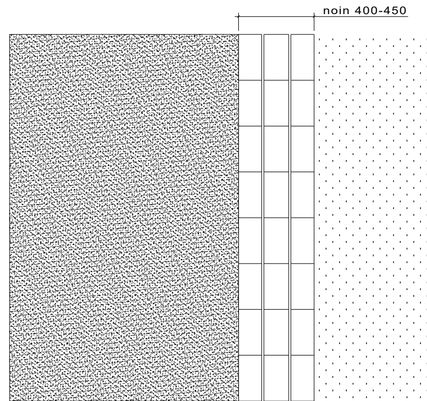
PUISTOKÄYTÄVÄ PÄÄLTÄ 1:20
