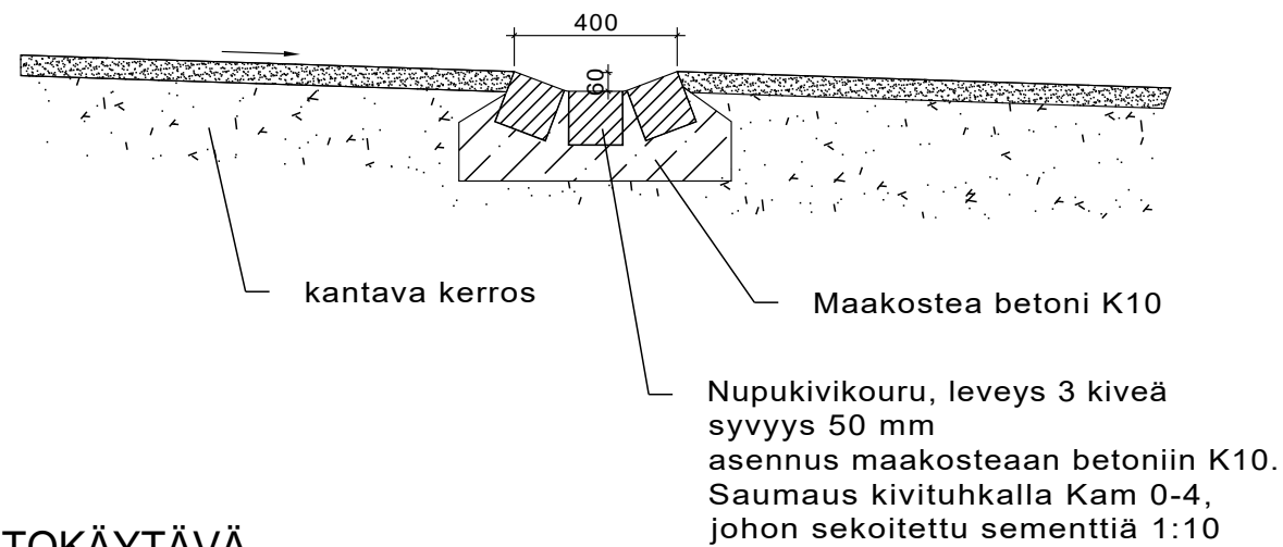
PUISTOKÄYTÄVÄ POIKKILEIKKAUS C-C 1:20
