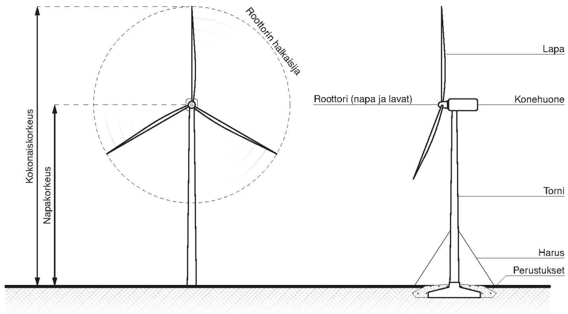
Kuva 7-1 Havainnekuva tuulivoimalasta
